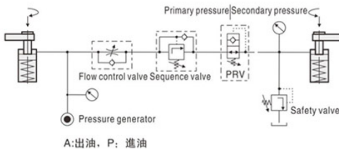
迴路圖 Circuit diagram
