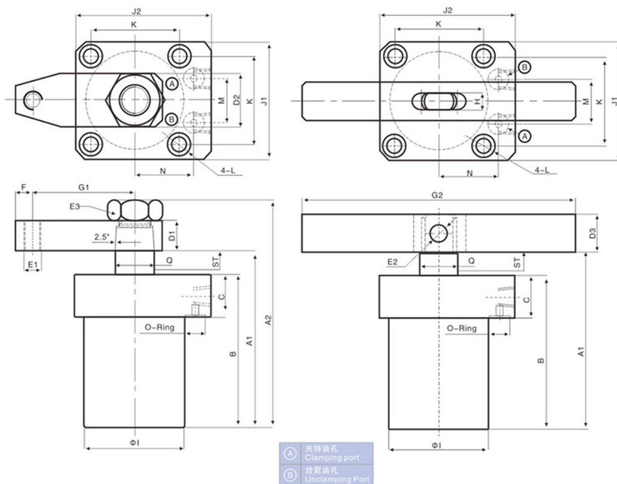
外形尺寸表 Dimension table
