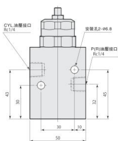
VEF-LT 配管型 ※附帶內部過濾器 (P、CYL油壓接口)
