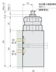
VEF-LT 配管型 ※附帶內部過濾器 (P、CYL油壓接口)
