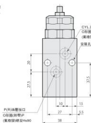
VEF-LT 配管型 ※附帶內部過濾器 (P、CYL油壓接口)
