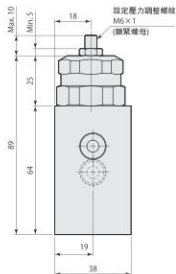
VEF-LT 配管型 ※附帶內部過濾器 (P、CYL油壓接口)
