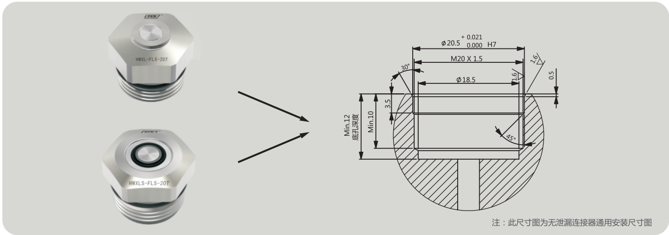
无泄漏连接器安装尺寸图：
