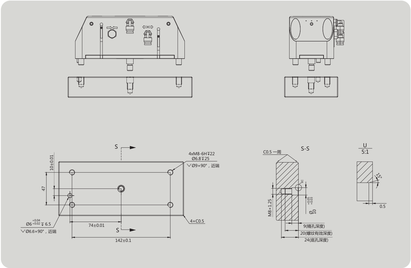
联轴器安装尺寸：
