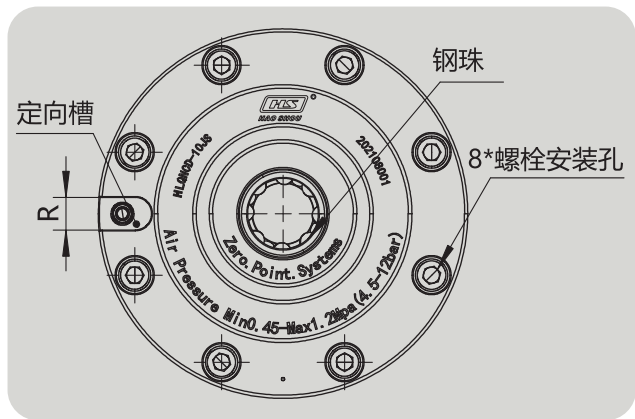
△ 外形尺寸图:
