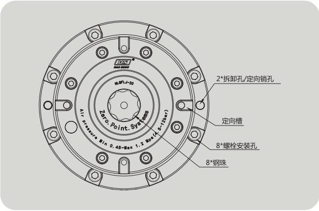
△ 尺寸图：
